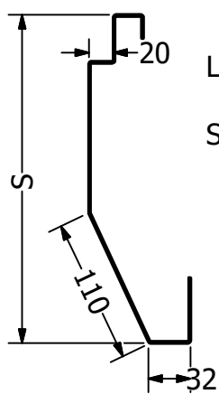
Dettaglio Battente
