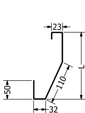
Dettaglio Montante
